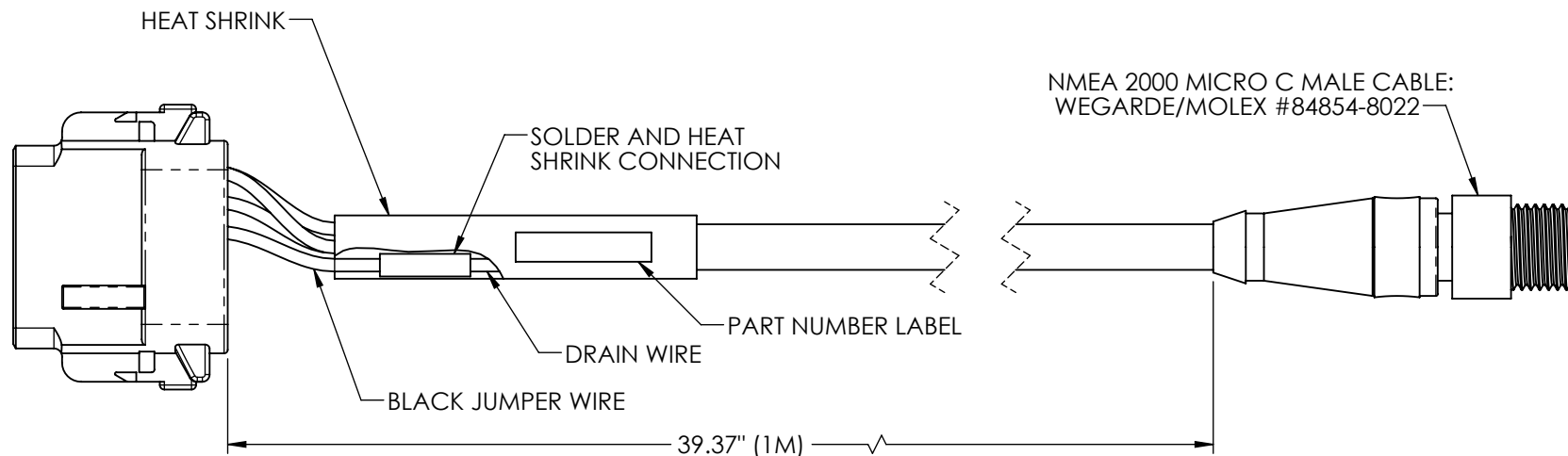
DEUTSCH DTM06-12SA
